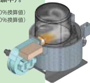
ラウンドNEOSの燃焼室構造 ▶ ※本図は、3Dによるイメージ画像ですので、実物とは異なる部分があります。
