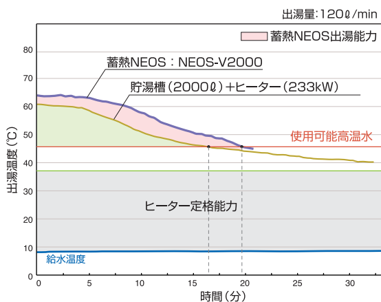
蓄熱NEOS 出湯特性比較
