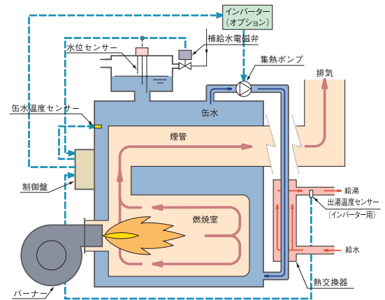
NEOSシステム構成
