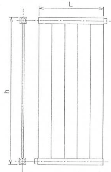
PHXV (縦型)
